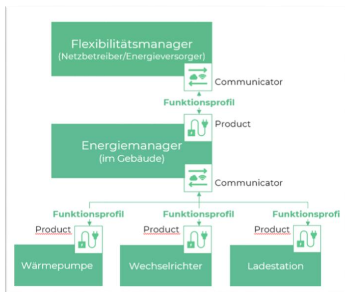
Abbildung 1: hierarchische Kommunikationsstruktur zur Veranschaulichung der SmartGridready-Begriffe
